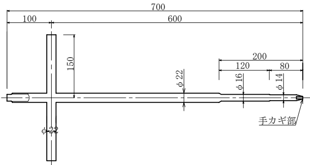
手カギ部詳細図
