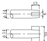
手カギ部詳細図
