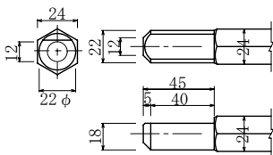
バール部詳細図
