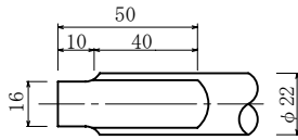
バール部詳細図
